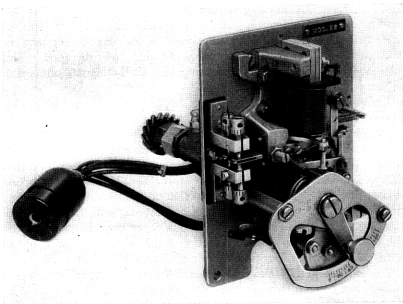
Fig. 6—Regenerator unit.
