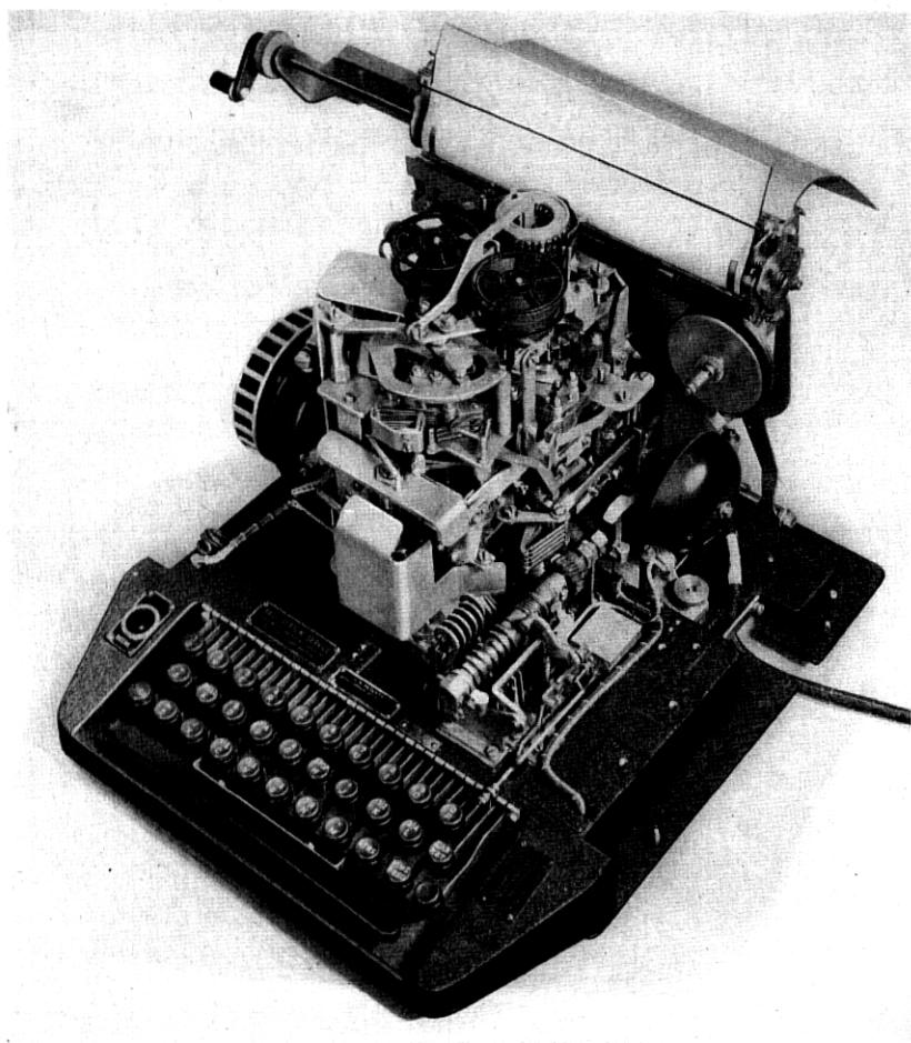
Fig. 7—No. 26 teletypewriter.
