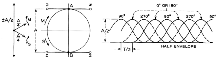
Fig. 7 — FM.
