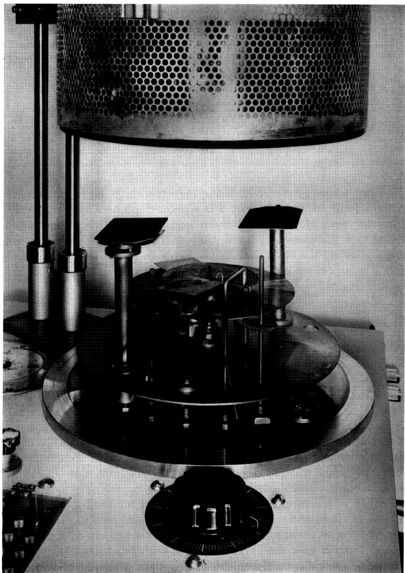
Fig. 14—Sputtering apparatus.
